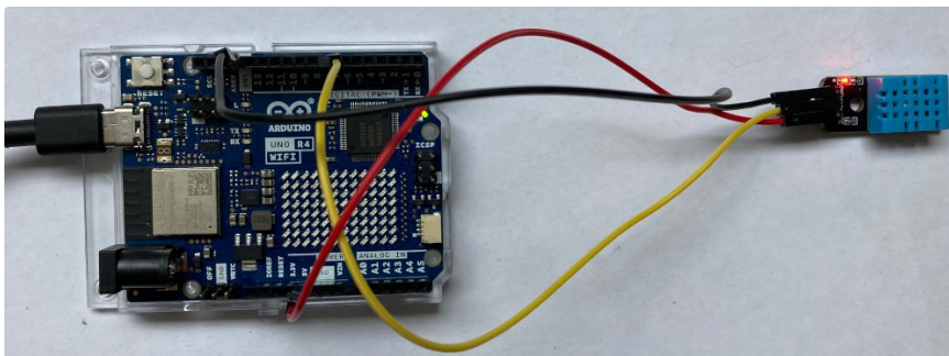
Arduino UNO R4 WiFi DHT11
